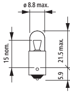
T4W
