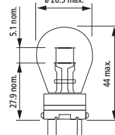
3157
