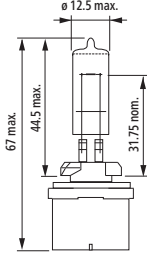
885, 893
