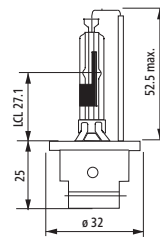
D2R
