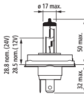
R2 Halogen
