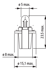
Bax 8,3d
