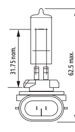
886, 894, 896
