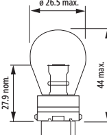
3156
