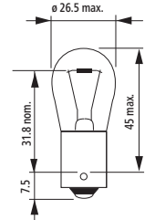
P(Y)21W
