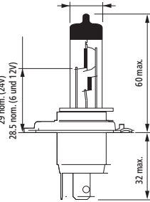
R2 Halogen
