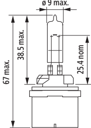
890
