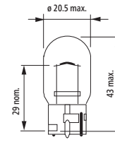
W(Y)21W
