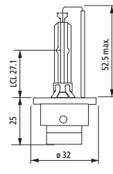
D2S, D4S
